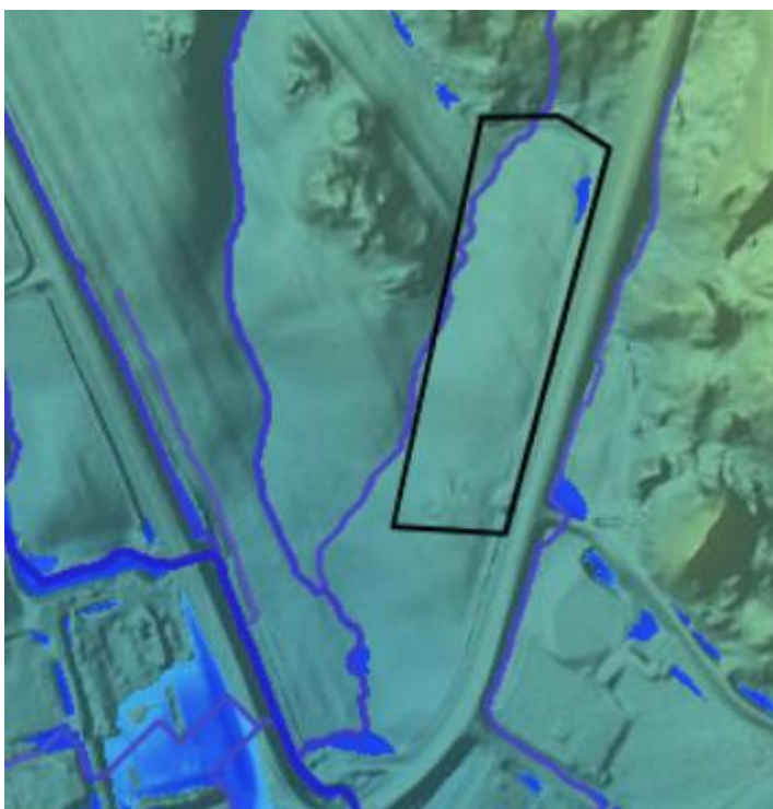
Figur 6: Skyfallsanalys i Scalgo. Källa: Scalgo Live 2020.
